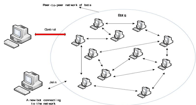
Fig. 5 P2P Botnet
